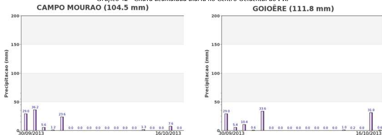
Gráfico 42 - Chuva acumulada diária no Centro Ocidental do PR.
