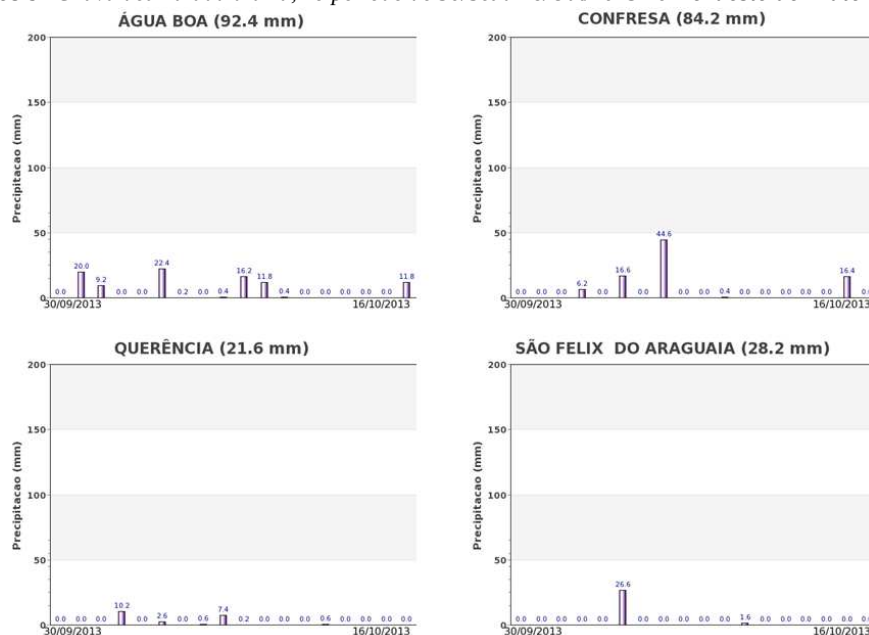
Gráficos 9- Chuva acumulada diária, no período de 30/Set a 16/Out/2013 no Nordeste do Mato Grosso.
