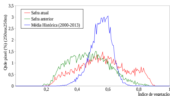
Gráfico 43- Quantificação de áreas agrícolas pelo valor do IV
