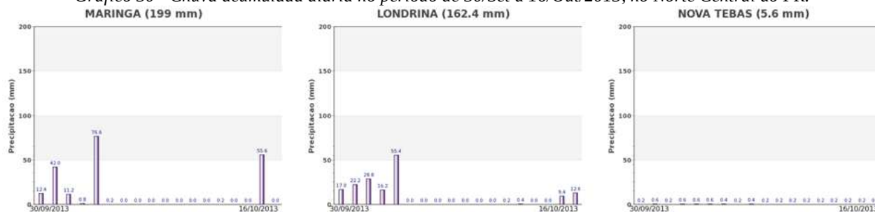
Gráfico 30 - Chuva acumulada diária no período de 30/Set a 16/Out/2013, no Norte Central do PR.
