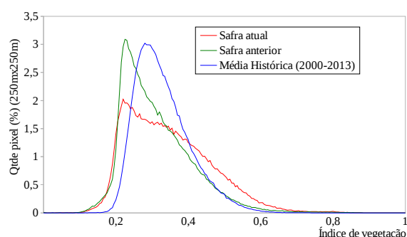
Gráfico 16- Quantificação de áreas pelo valor do IV
