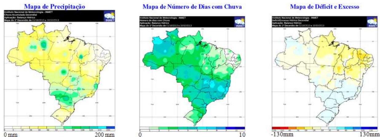
Mapa 33 – Precipitação, número de dias com chuva e déficit/excesso hídrico no período de 1º a 10 de outubro/2013.
