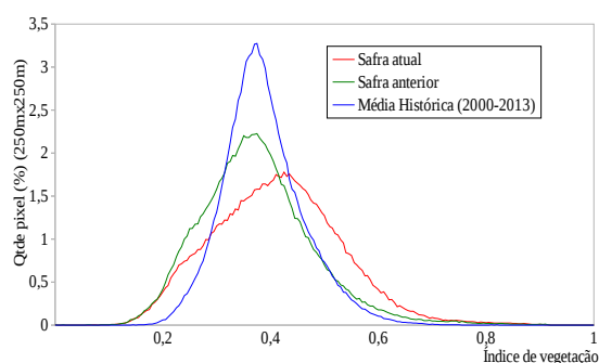
Gráfico 46- Quantificação de áreas pelo valor do IV
