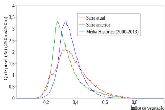
Gráfico 7- Quantificação de áreas pelo valor do IV
