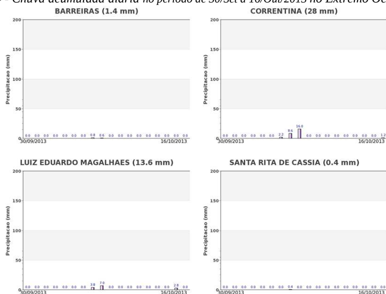
Gráfico 24 - Chuva acumulada diária no período de 30/Set a 16/Out/2013 no Extremo Oeste Baiano.
