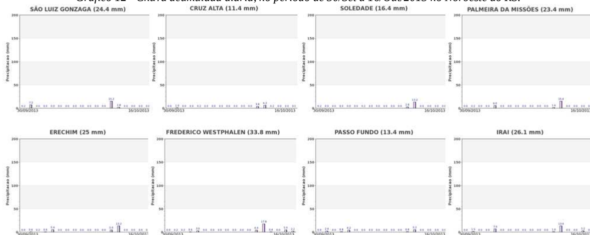
Gráfico 12 - Chuva acumulada diária, no período de 30/Set a 16/Out/2013 no Noroeste do RS.
