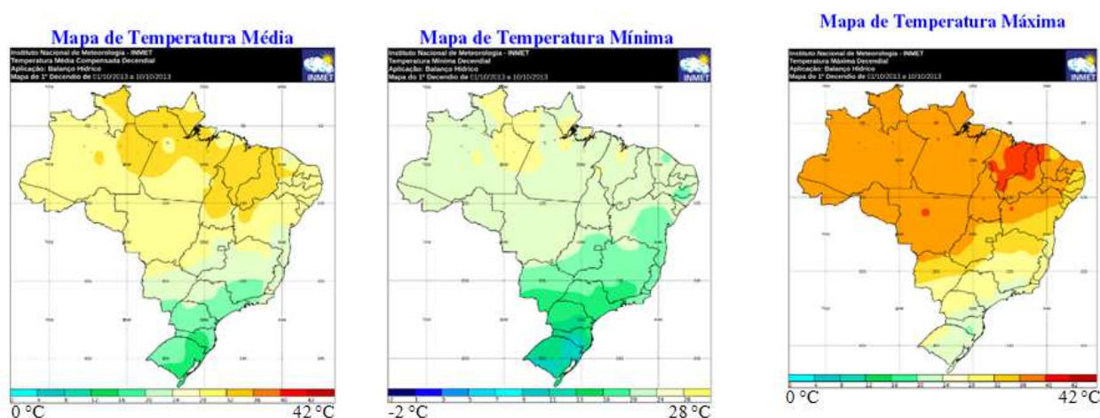
Mapa 34 – Temperaturas média, mínima e máxima no período de 1º a 10 de outubro/2013.
