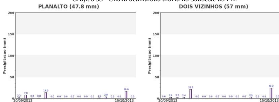
Gráfico 33 - Chuva acumulada diária no Sudoeste do PR.
