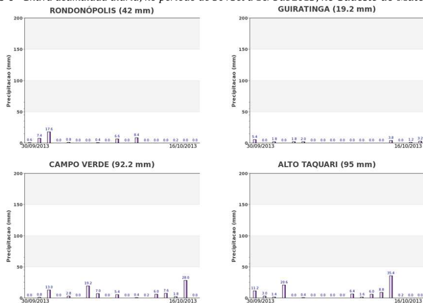
Gráficos 6- Chuva acumulada diária, no período de 30/Set a 16/Out/2013, no Sudeste do Mato Grosso.
