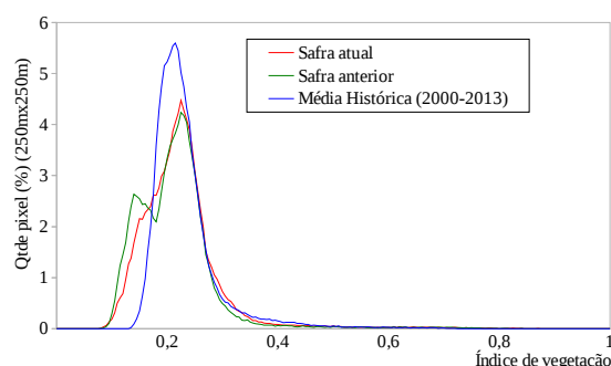
Gráfico 22- Quantificação de áreas pelo valor do IV
