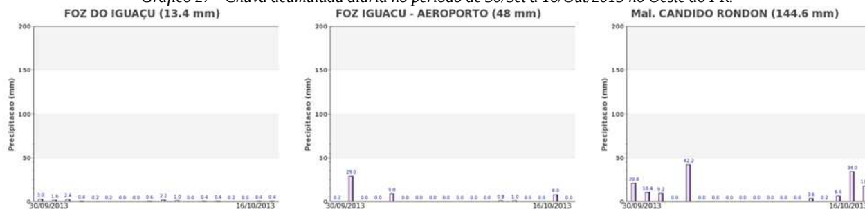
Gráfico 27 - Chuva acumulada diária no período de 30/Set a 16/Out/2013 no Oeste do PR.
