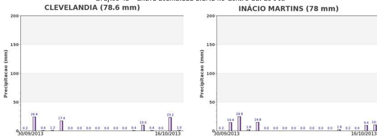
Gráfico 45 - Chuva acumulada diária no Centro-Sul do PR.
