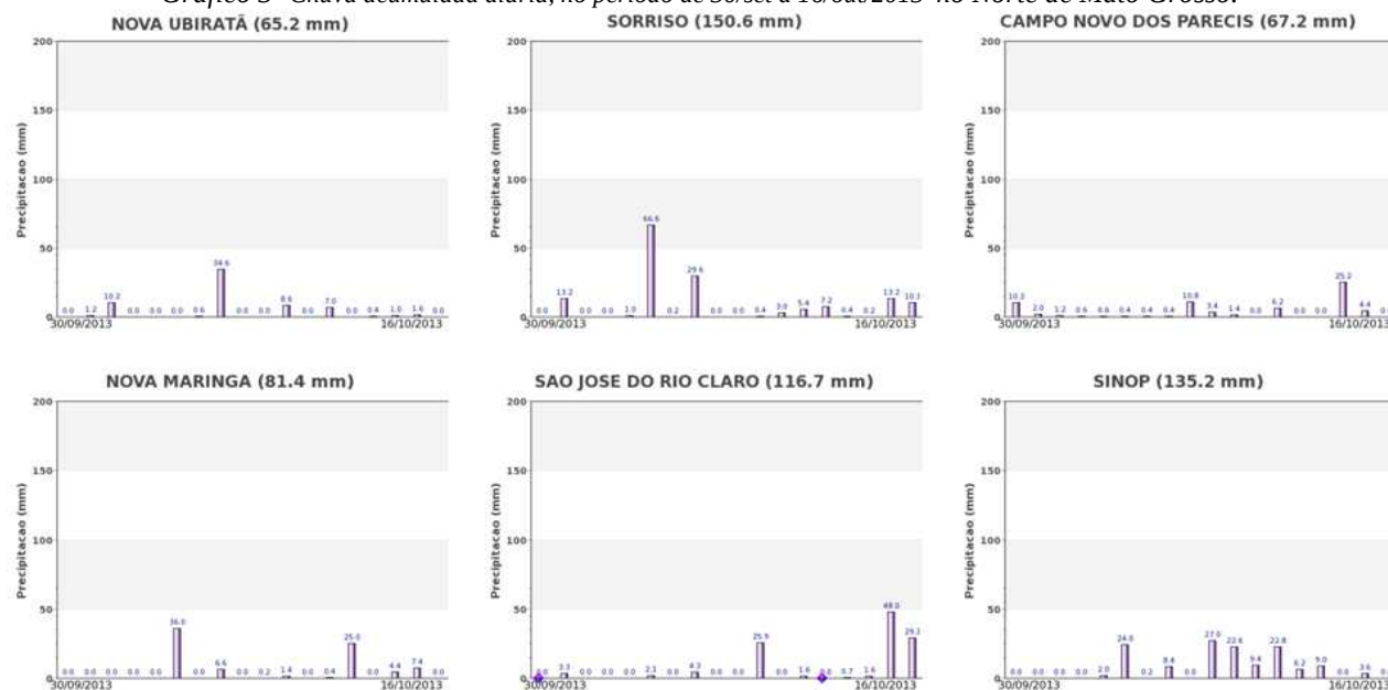
Gráfico 3- Chuva acumulada diária, no período de 30/set a 16/out/2013 no Norte de Mato Grosso.
