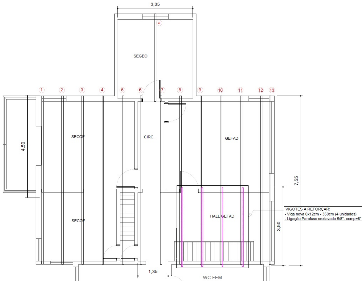
Figura 2 : Planta vigas a imunização e localização do reforço do madeiramento
