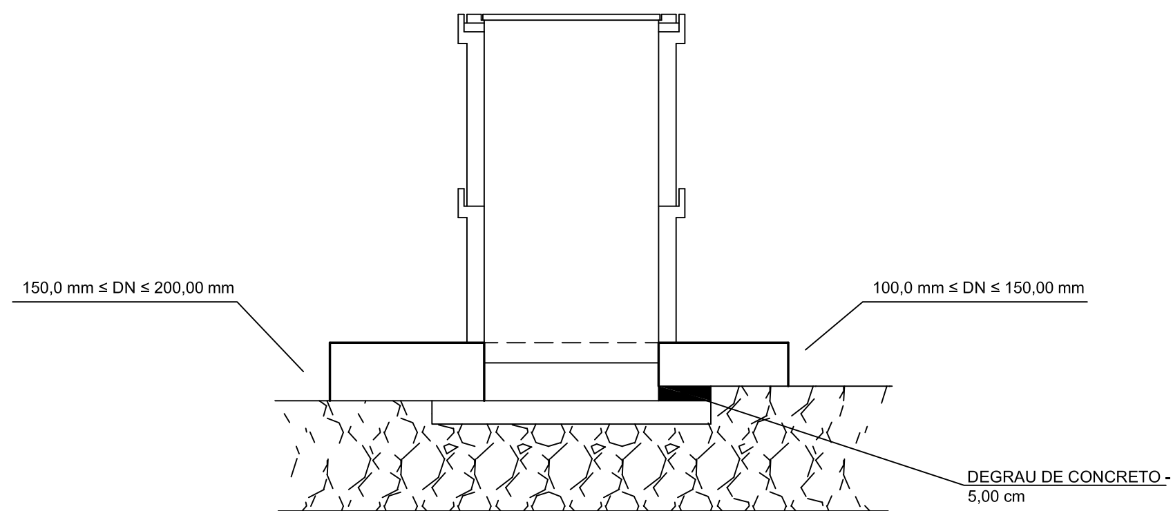
DETALHE - DEGRAU DA CAIXA DE PASSAGEM
