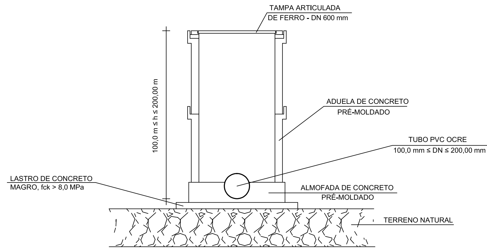
CAIXA DE PASSAGEM
