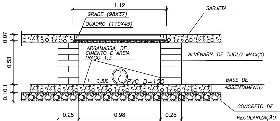
CORTE D-D
