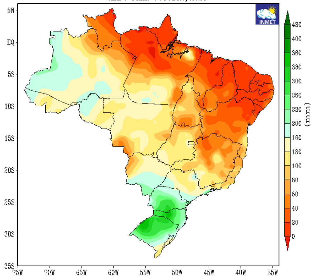
PRECIPITAÇÃO TOTAL PREVISTA (mm) ATUALIZAÇÃO - SETEMBRO/2023 VALIDO PARA OUTUBRO/2023
