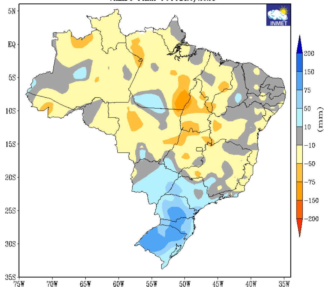
PREVISÃO DE ANOMALIAS DE PRECIPITAÇÃO (mm) ATUALIZAÇÃO - SETEMBRO/2023 VALIDO PARA OUTUBRO/2023
