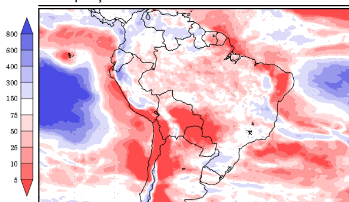
Precipitação Percentual Acima da Normal
