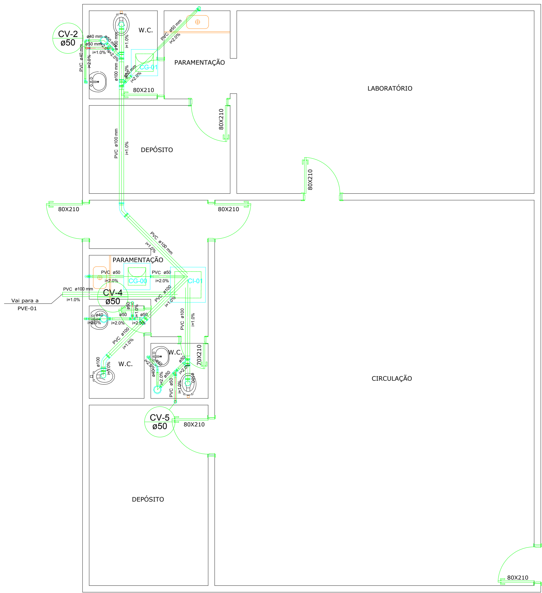
SANITÁRIOS GRANELEIRO BUFFALO ESCALA : 1/50
