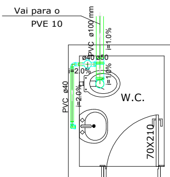
SANITÁRIO GUARITA ESCALA : 1/50
