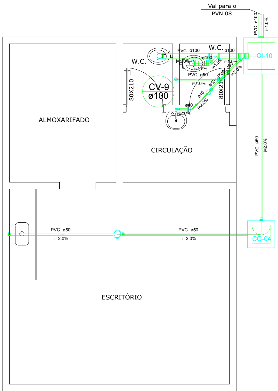
APOIO ARMAZÉNS CONVENCIONAIS 01/02 ESCALA : 1/50
