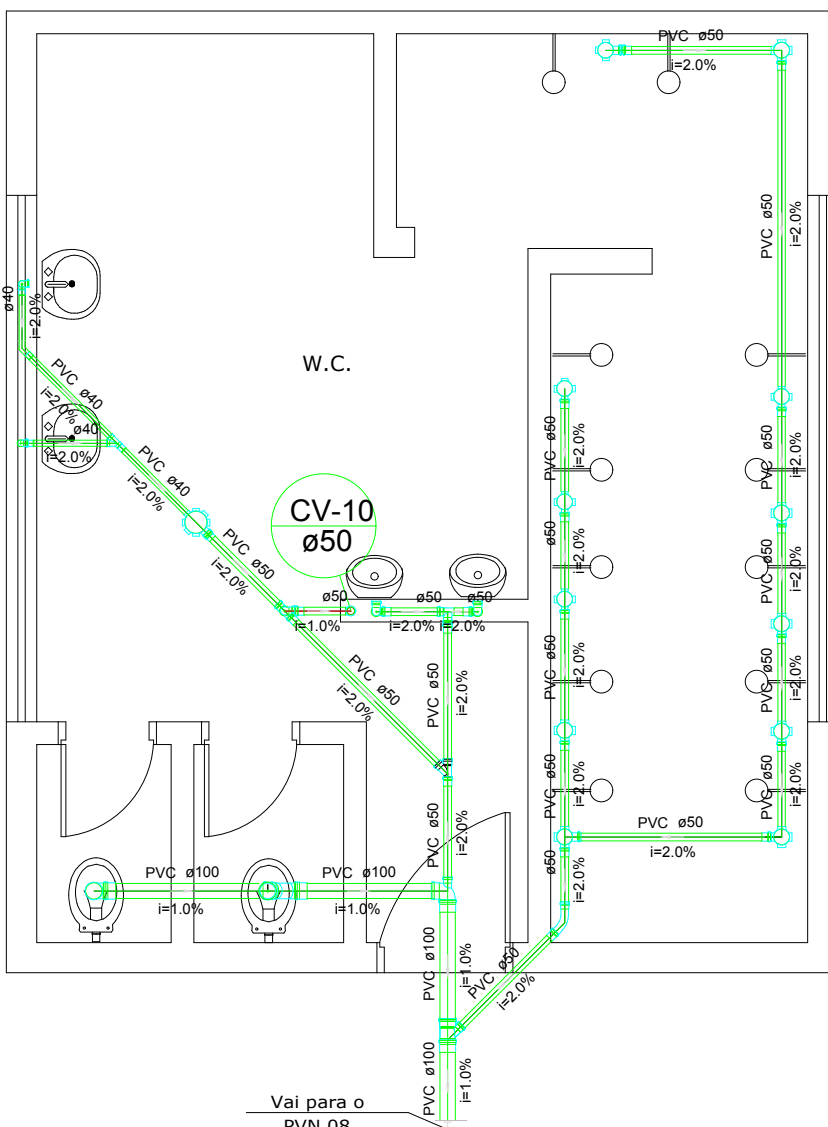
APOIO ARMAZÉNS CONVENCIONAIS 02/02 ESCALA : 1/50
