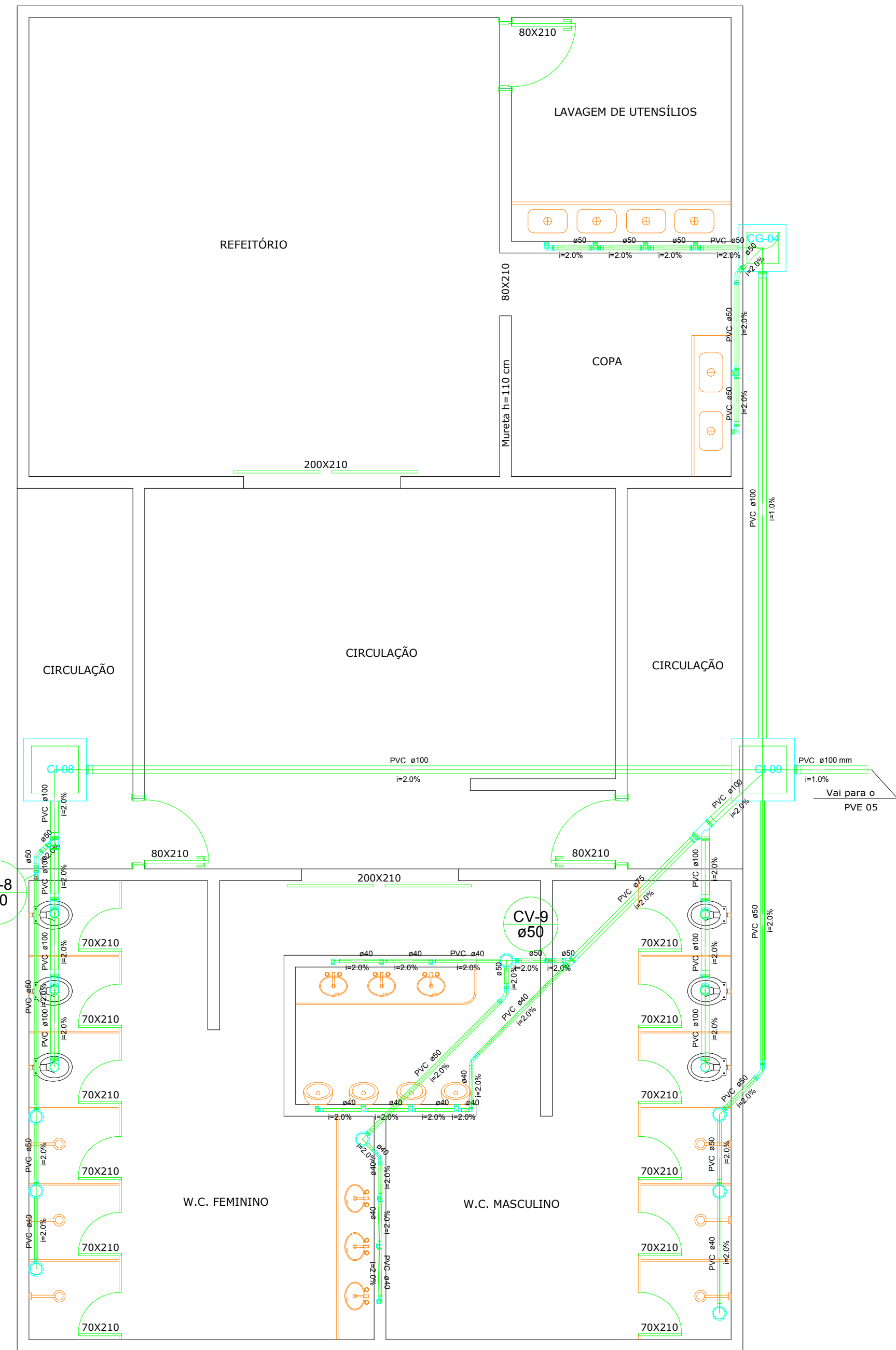
VESTIÁRIOS E REFEITÓRIO ESCALA : 1/50
