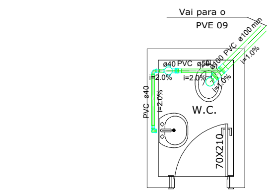
SANITÁRIO PRÉ-CLASSIFICAÇÃO ESCALA : 1/50
