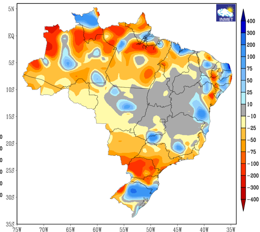
ANOMALIA DE PRECIPITAÇÃO VALIDO PARA JUNHO DE 2024
