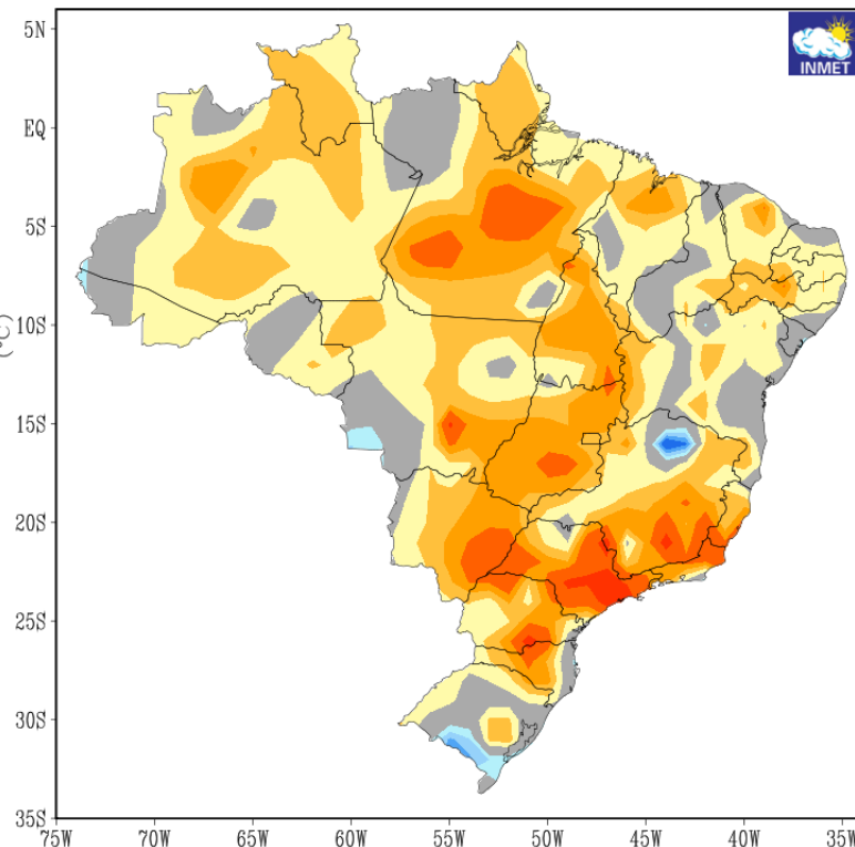
ANOMALIAS DE TEMPERATURAS MÉDIAS VÁLIDO PARA MAIO DE 2024 CLIMATOLOGIA DE REFERÊNCIA: 1981-2010
