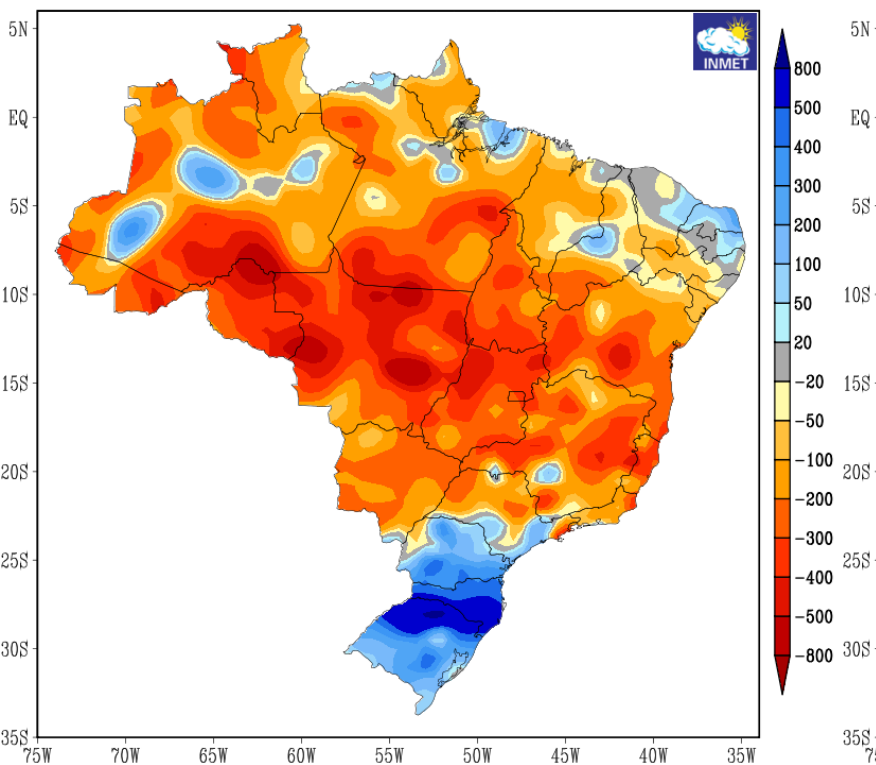
ANOMALIA DE PRECIPITAÇÃO TRIMESTRAL VALIDO PARA OUTUBRO, NOVEMBRO, DEZEMBRO DE 2023
