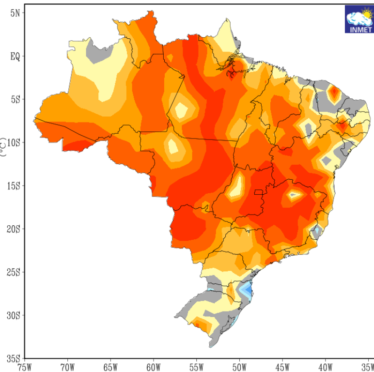
ANOMALIAS DE TEMPERATURAS MEDIAS VALIDO PARA NOVEMBRO DE 2023 CLIMATOLOGIA DE REFERENCIA:1981-2010
