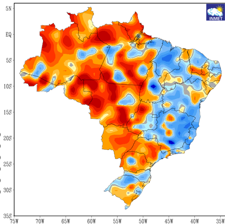
ANOMALIA DE PRECIPITAÇÃO TRIMESTRAL VALIDO PARA JANEIRO, FEVEREIRO, MARÇO DE 2024
