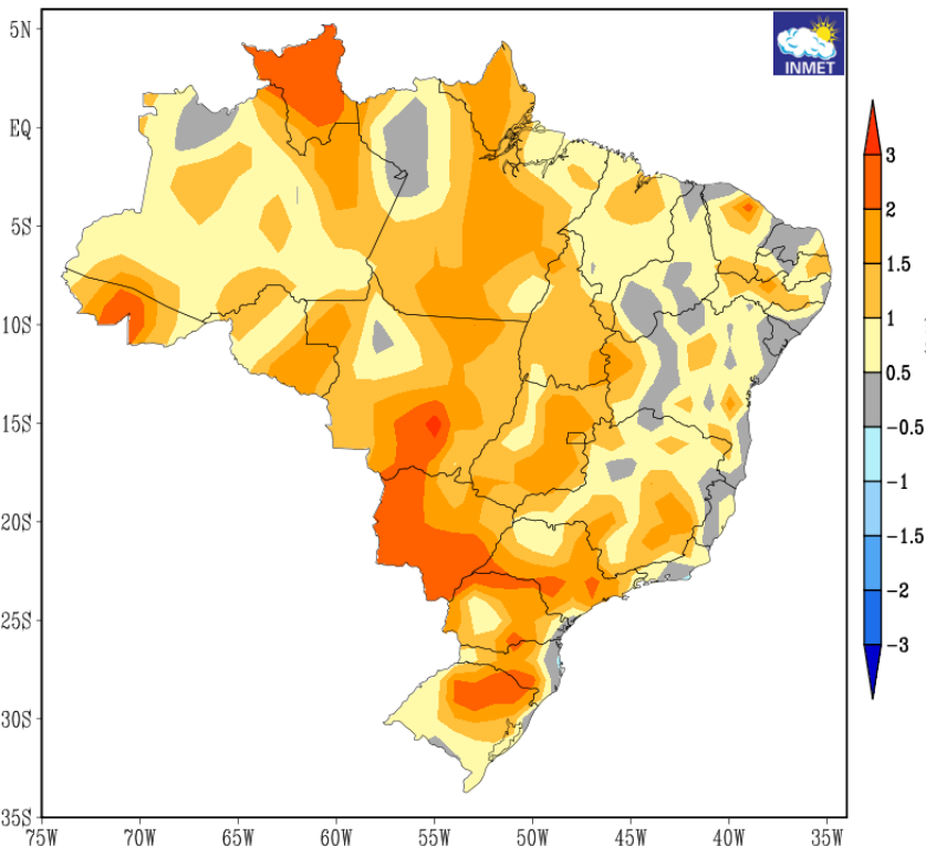
ANOMALIAS DE TEMPERATURAS MÉDIAS VÁLIDO PARA ABRIL DE 2024 CLIMATOLOGIA DE REFERÊNCIA: 1981-2010
