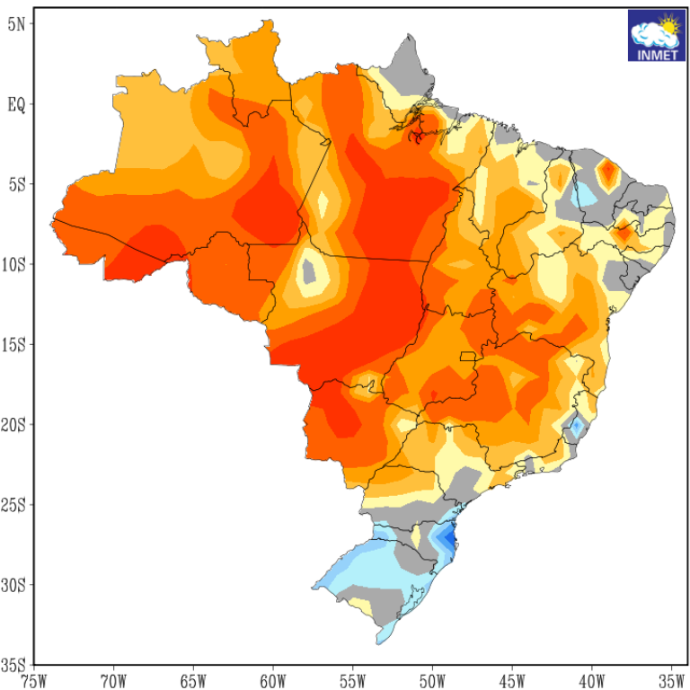
ANOMALIAS DE TEMPERATURAS MEDIAS VALIDO PARA OUTUBRO DE 2023 CLIMATOLOGIA DE REFERENCIA:1981-2010
