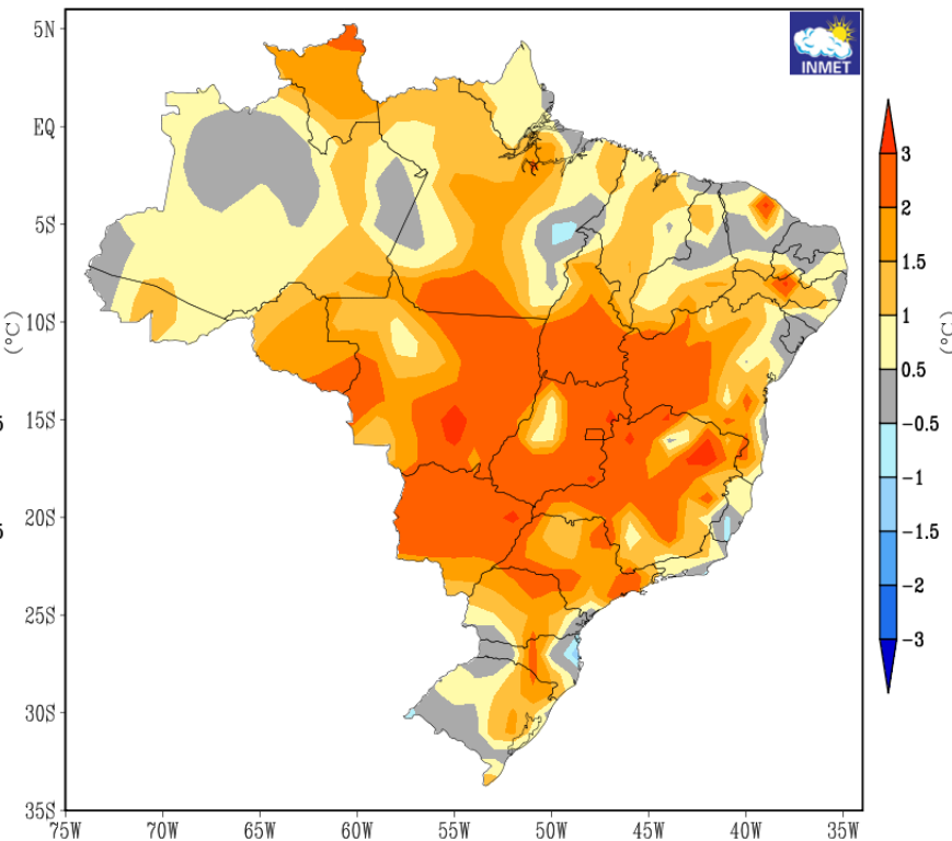
ANOMALIAS DE TEMPERATURAS MEDIAS VALIDO PARA DEZEMBRO DE 2023 CLIMATOLOGIA DE REFERENCIA:1981-2010
