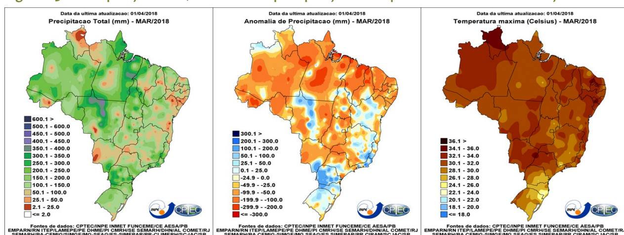
Figura 29 – Precipitação total, anomalia de precipitação e temperatura máxima em março de 2018
