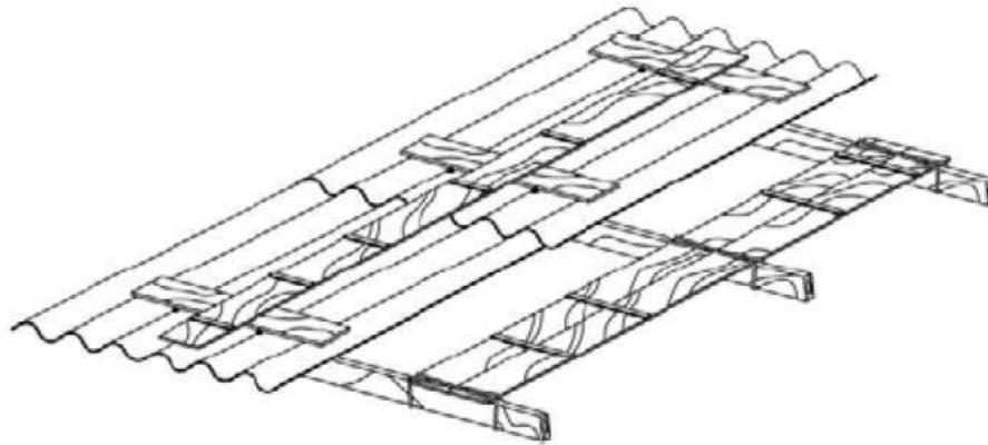
Tábuas para movimentação e distribuição de peso
