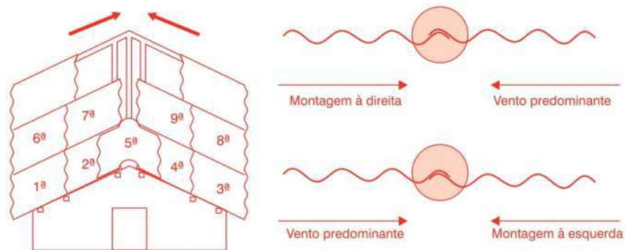
Sentido da montagem das telhas onduladas
