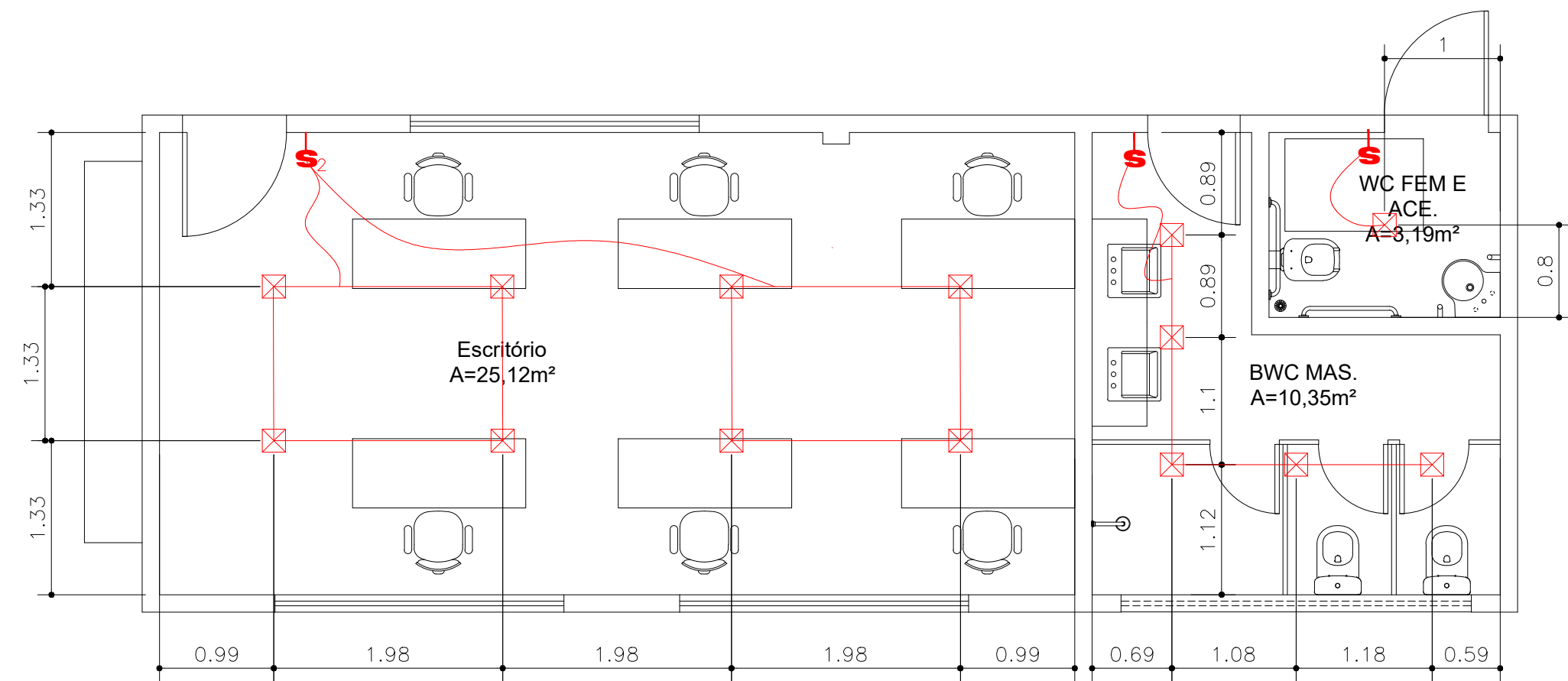
LUMINOTÉCNICO ESCALA 1/50
