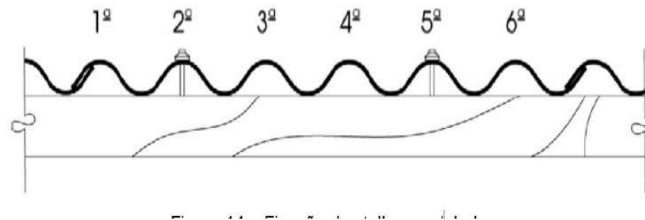
Fixação das telhas onduladas nas ondas altas;
