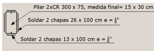
Figura 02: Detalhamento do reforço dos pilares
