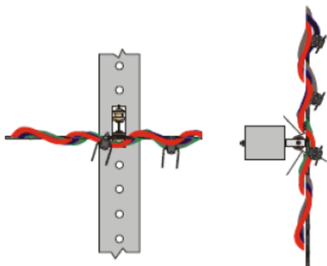
Figura 02: Amarração da rede Multiplexada (Estrutura S1)
